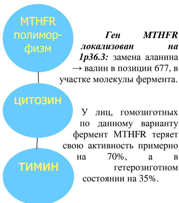
Рис. 2. Метилирование ДНК
